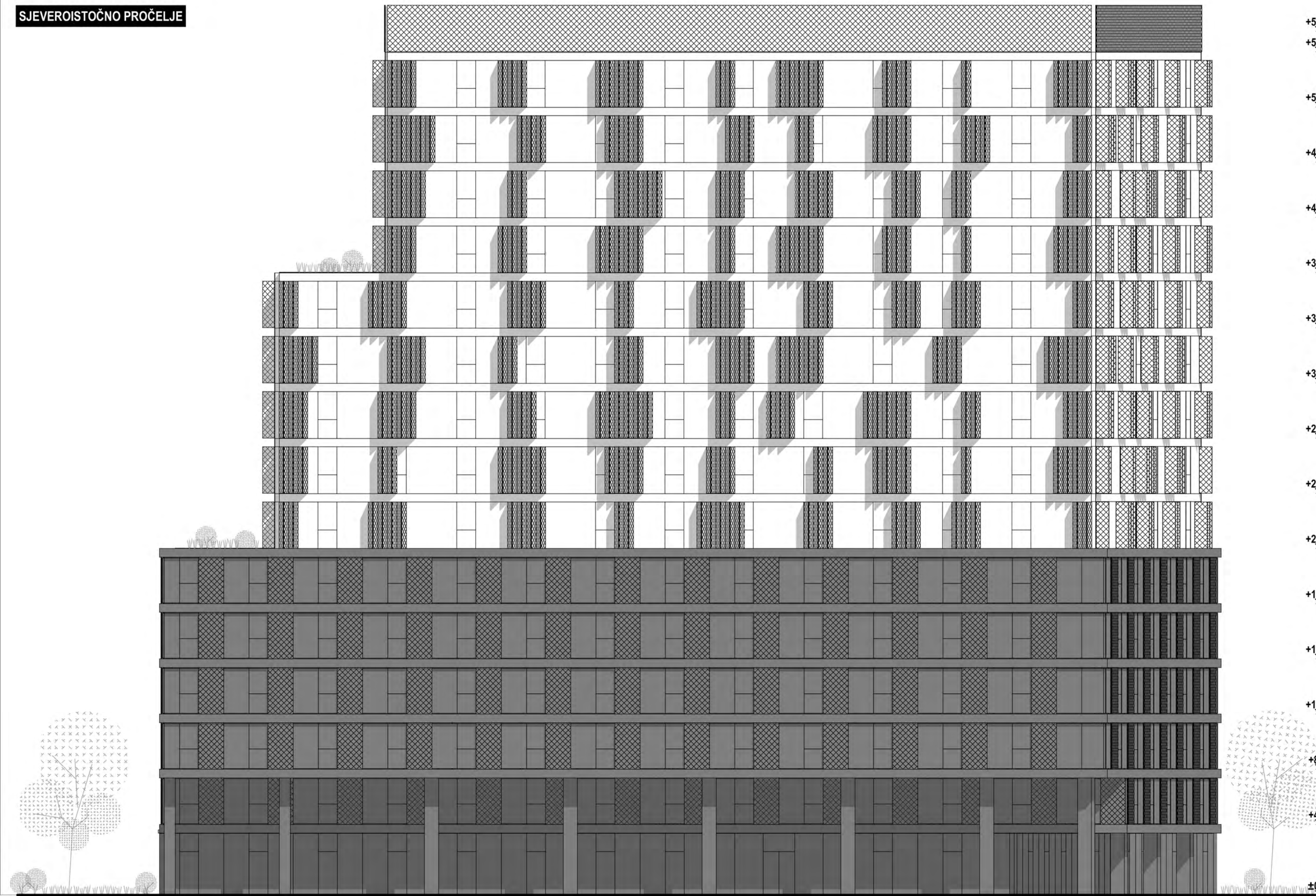
SJEVEROISTOČNO PROČELJE
