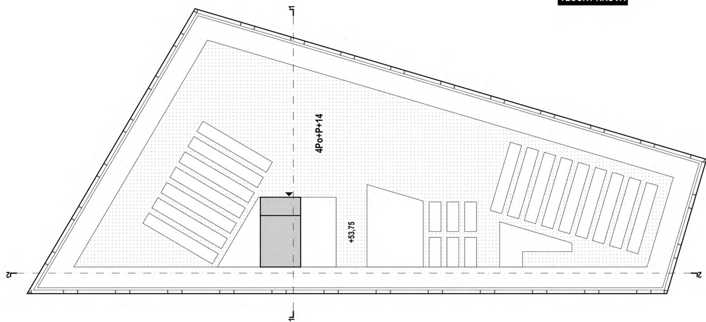
TLOCRT KROVA
