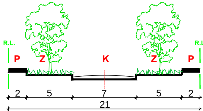
PRESJEK A-A
