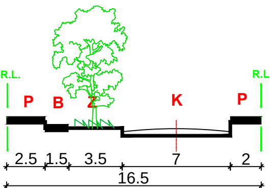
PRESJEK D-D
