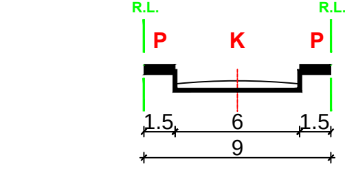
PRESJEK E-E
