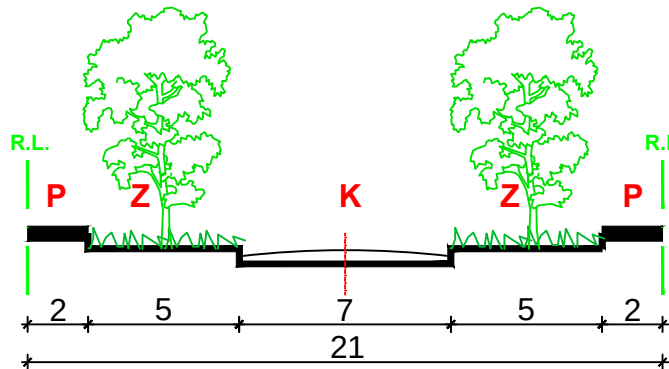
PRESJEK A-A
