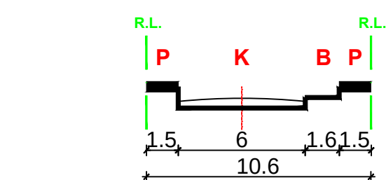
PRESJEK E1-E1
