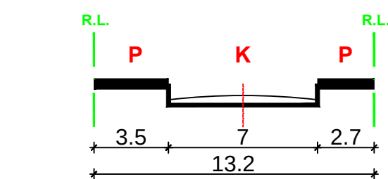
PRESJEK B-B
