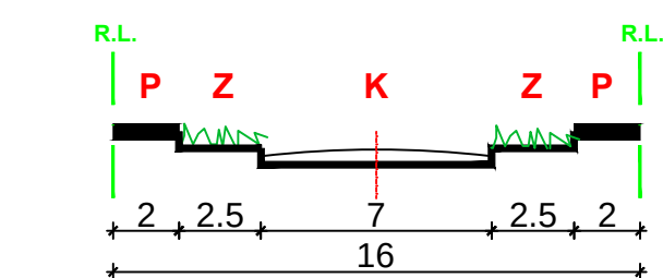
PRESJEK B1-B1
