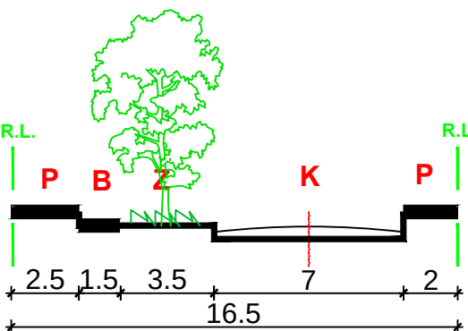
PRESJEK D-D
