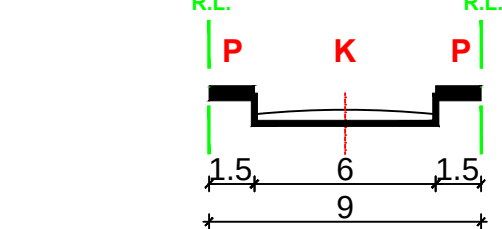
PRESJEK E-E
