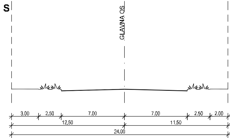
PRESJEK 5-5
