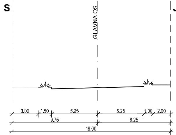
PRESJEK 4-4
