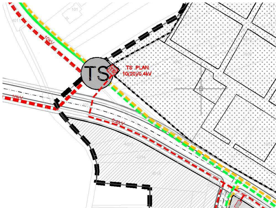
Prikaz trafostanice na zapadnom dijelu obuhvata Plana
