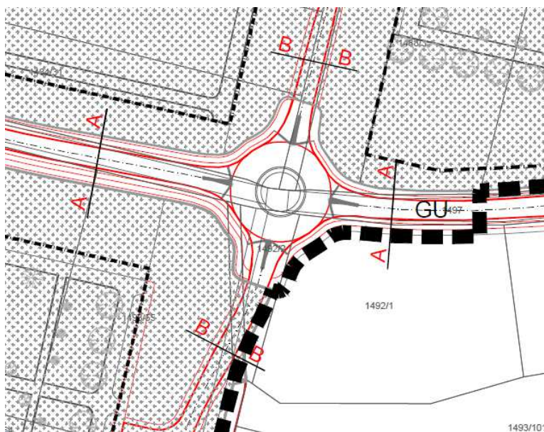
Prikaz planiranog kružnog raskrižja
