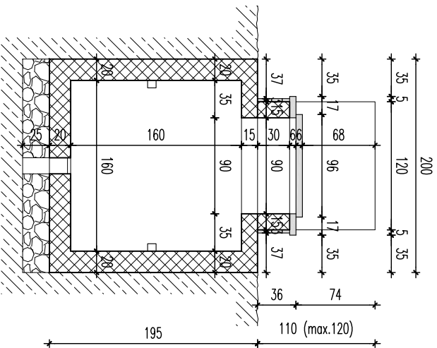
poprečni presjek
