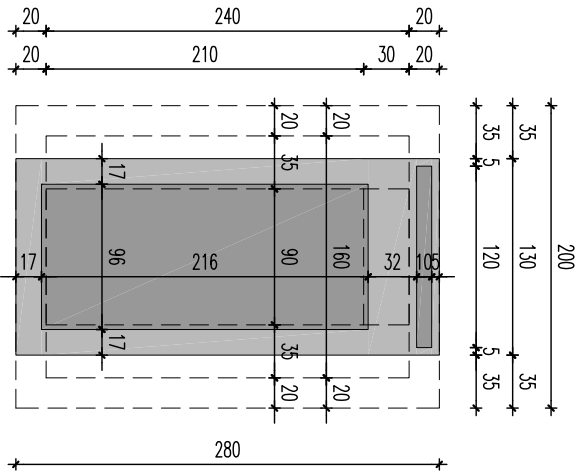
tllocrt
