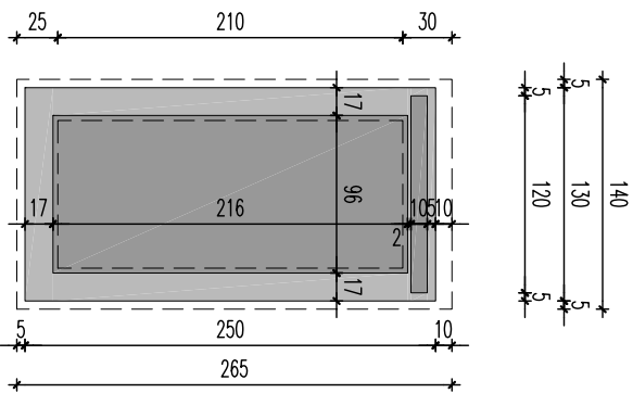
tllocrt
