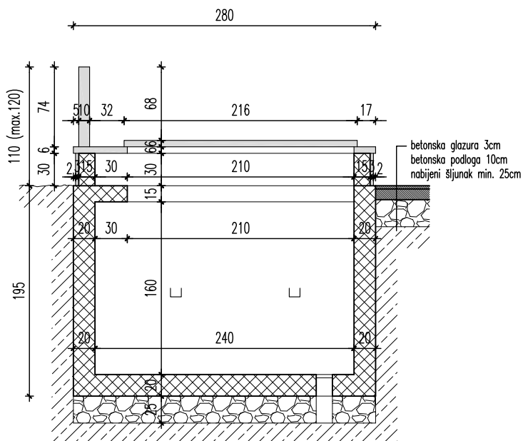
uzdužni presjek
