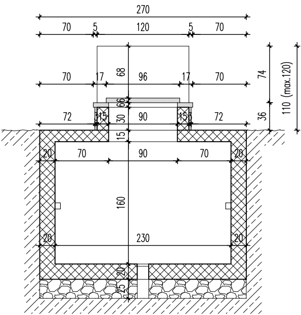
poprečni presjek
