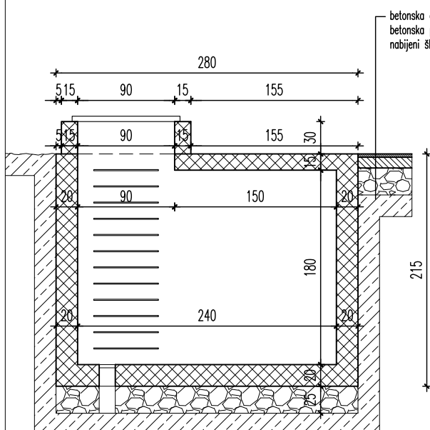
uzdužni presjek
