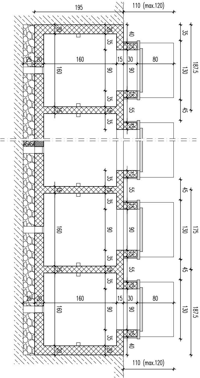
poprečni presjek
