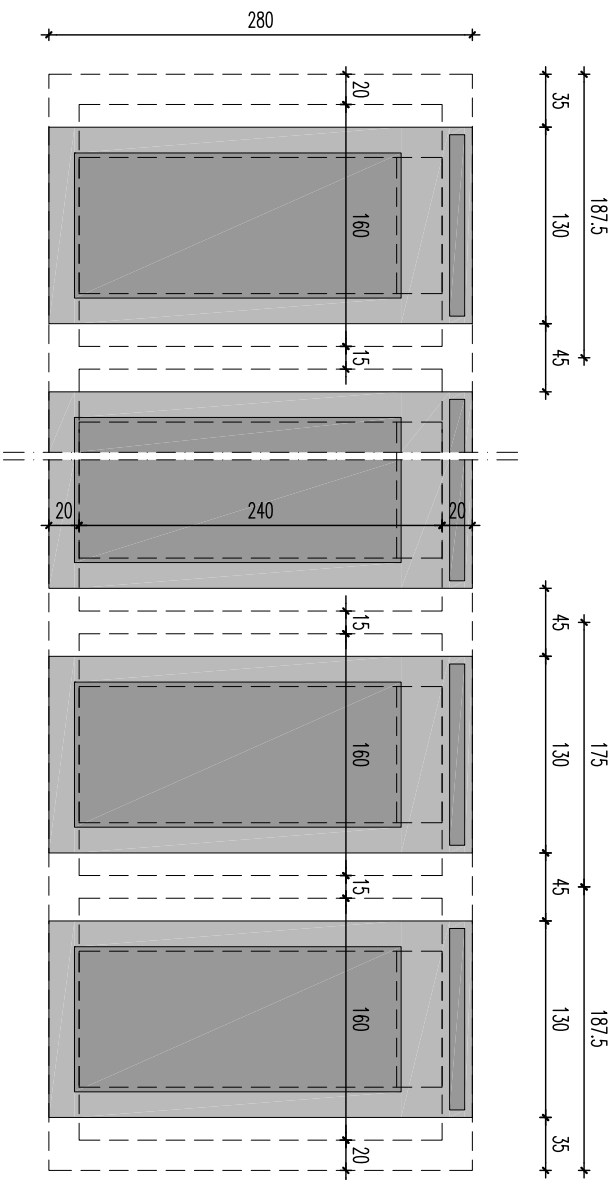
tllocrt
