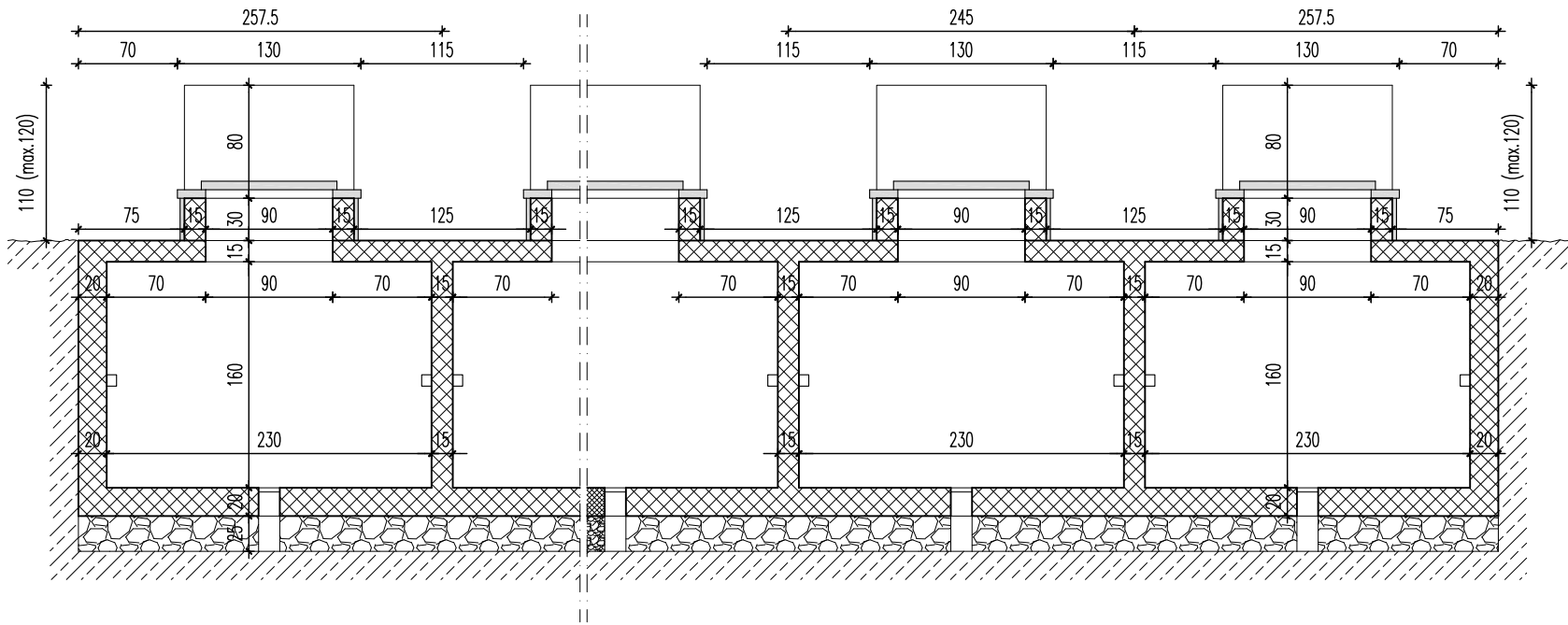
poprečni presjek
