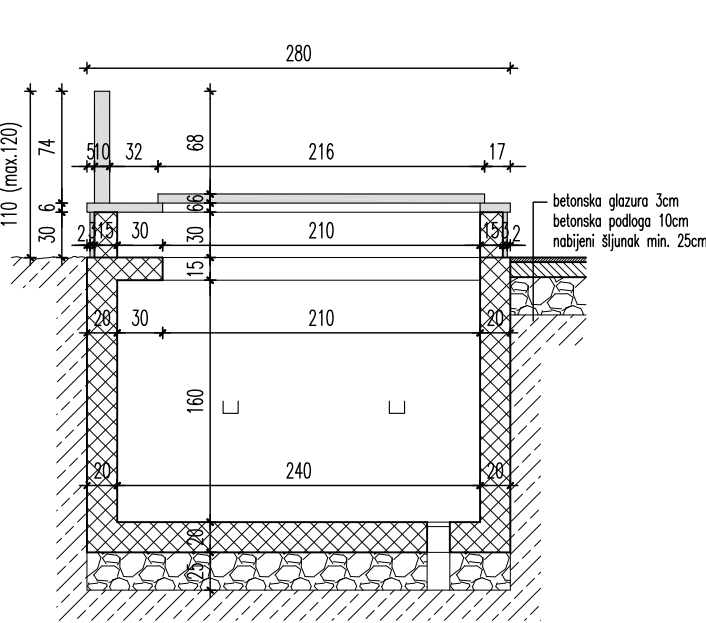
uzdužni presjek
