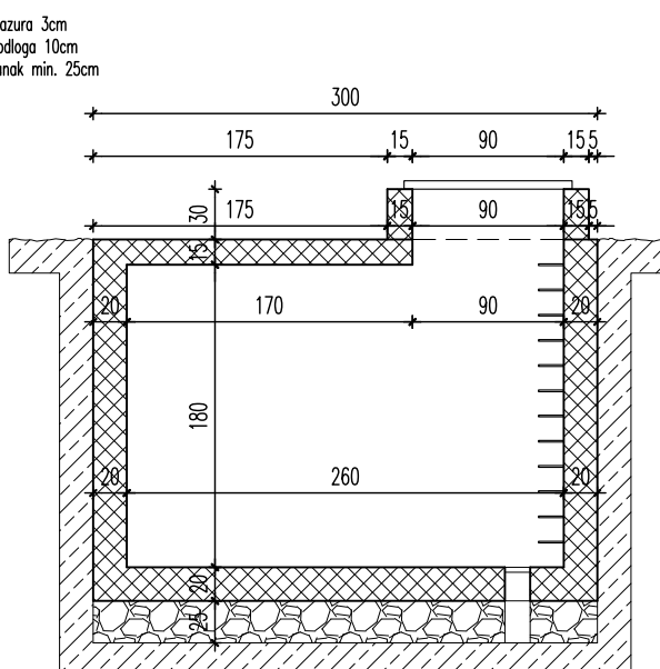
poprečni presjek
